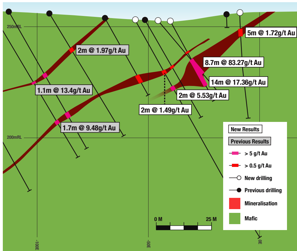
Lord Percy Oblique Section
