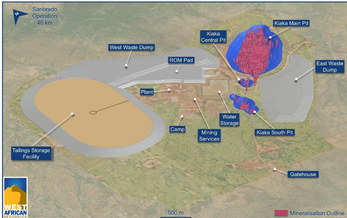
Kiaka schematic layout
